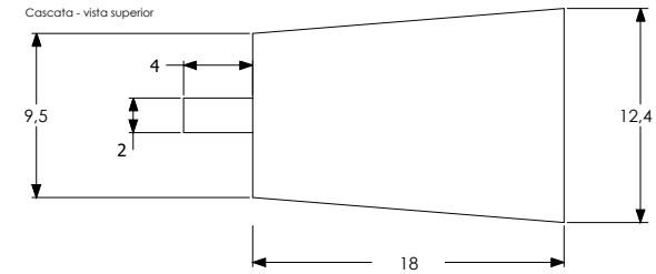
Cascata - vista superior
