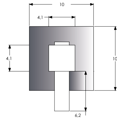
Misturador e canopla - vista frontal
